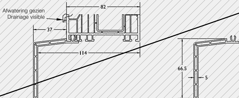
Dorpel ■ Seuil 7788
