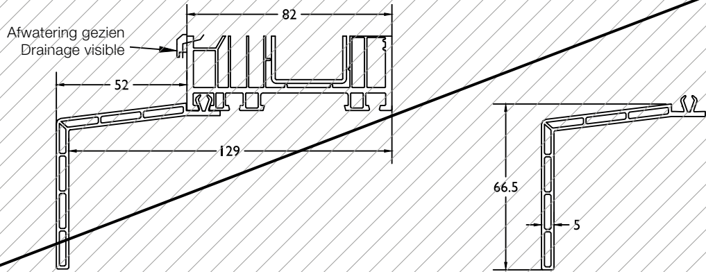
Dorpel ■ Seuil 7607
