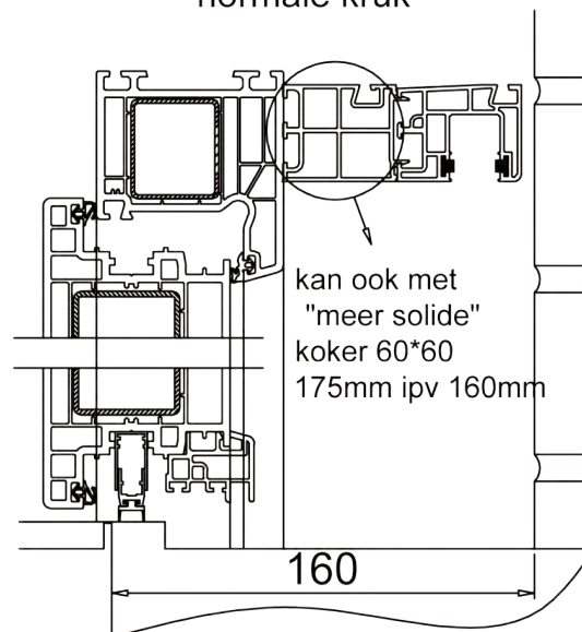
Deur ct70 met rolluik met doorlopende normale kruk
