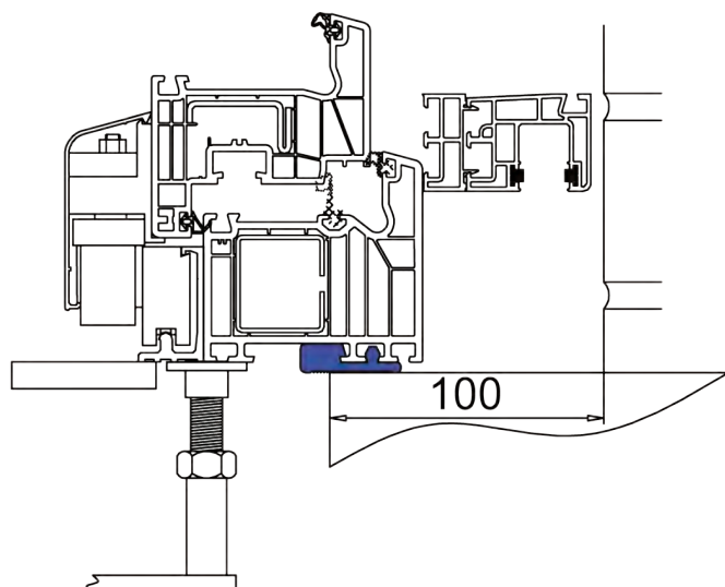
kipschuif Thermo6 met rolluik en/of dunne schuifhor
