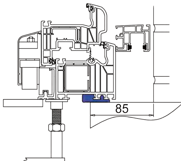
kipschuif Thermo6 met rolluik
