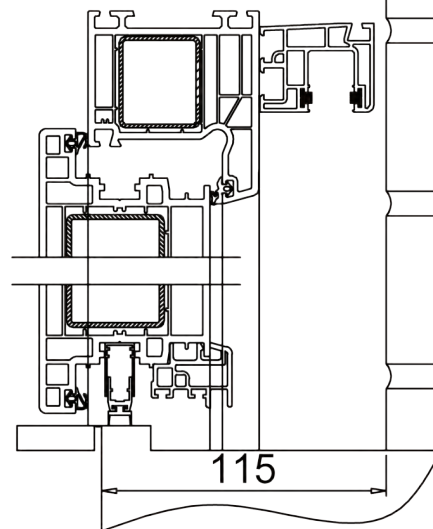
Deur CT70 met rolluik
