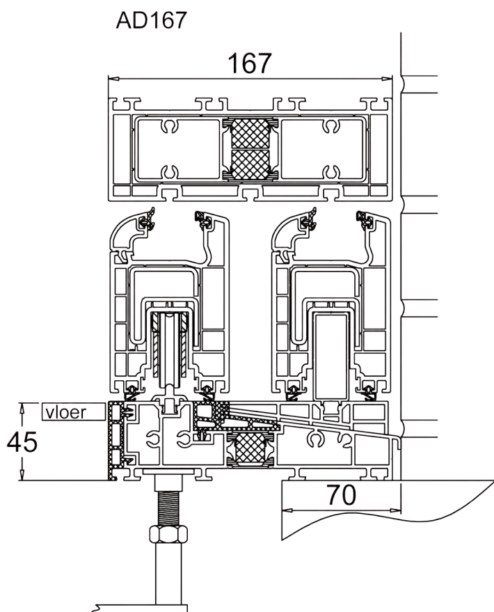
AD167 met rolluik en dunne schuifhor
