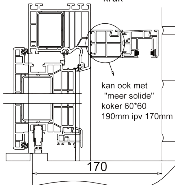
Deur Thermo6 met rolluik met doorlopende normale kruk
