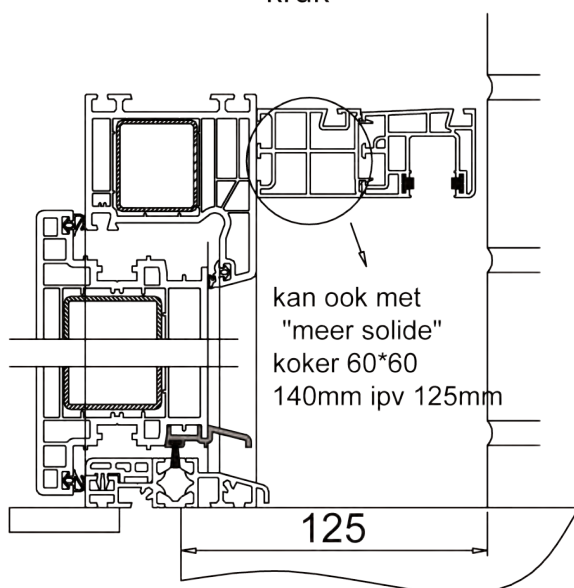
Deur CT70 met rolluik met doorlopende normale kruk
