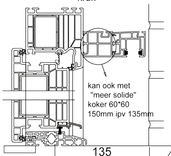
Deur Thermo6 met rolluik met doorlopende normale kruk
