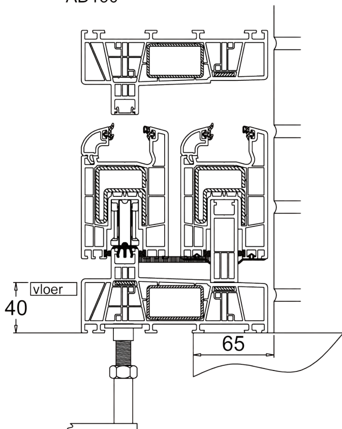
AD150 met rolluik en dunne schuifhor
