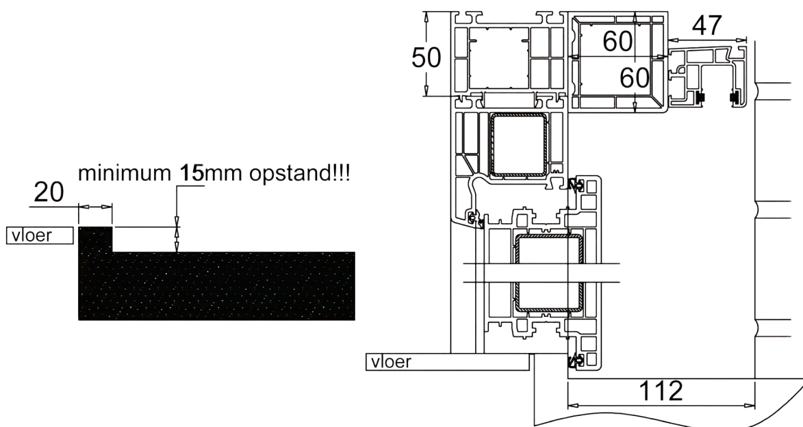
Deur CT70 met rolluik
