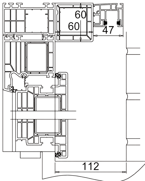
Deur Thermo6 met rolluik
