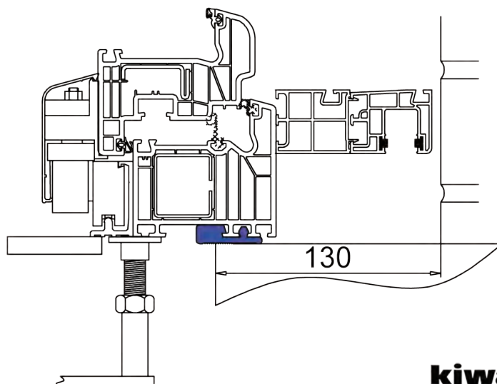
kipschuif Thermo6 met rolluik met normale schuifhor
