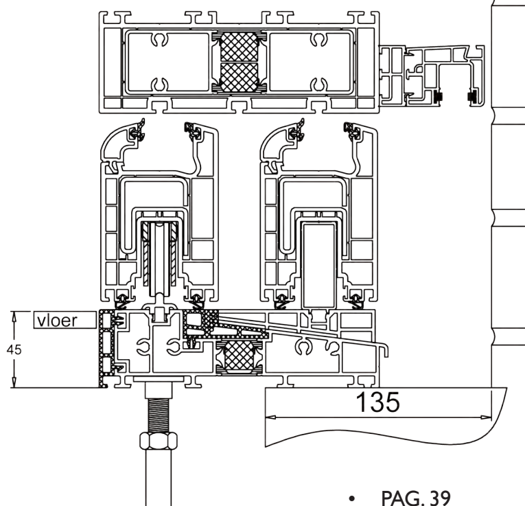
AD167 met rolluik en dunne schuifhor
