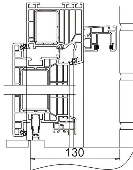
Deur Thermo6 met rolluik
