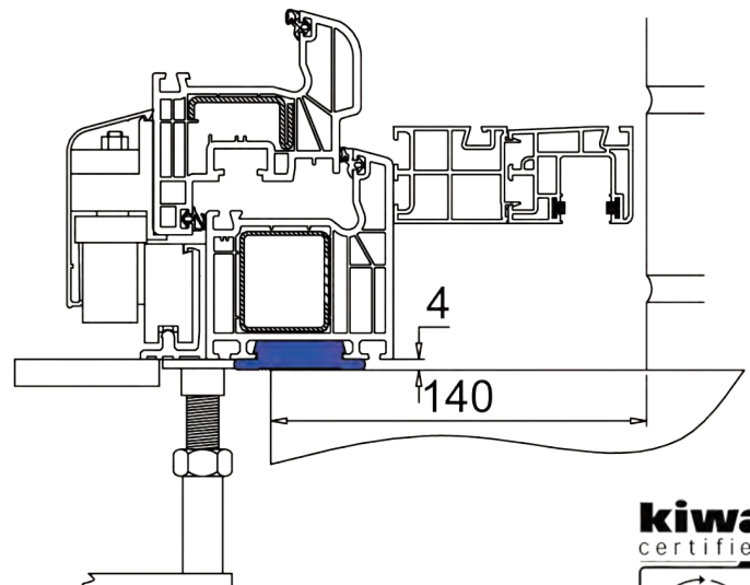
kipschuif CT70 met rolluik met normale schuifhor
