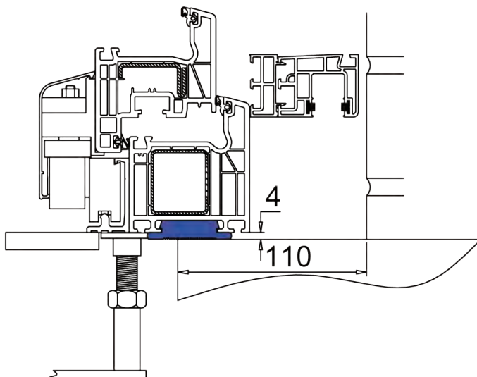
kipschuif CT70 met rolluik en/of dunne schuifhor
