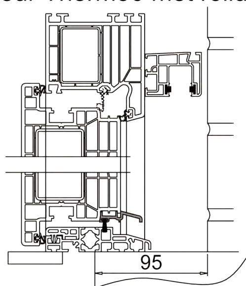
Deur Thermo6 met rolluik
