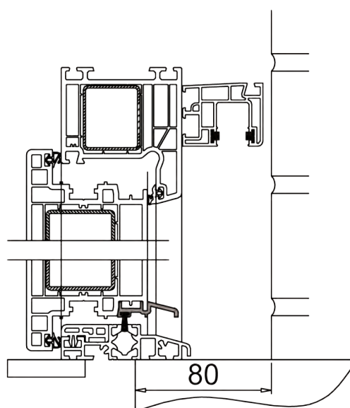
Deur CT70 met rolluik
