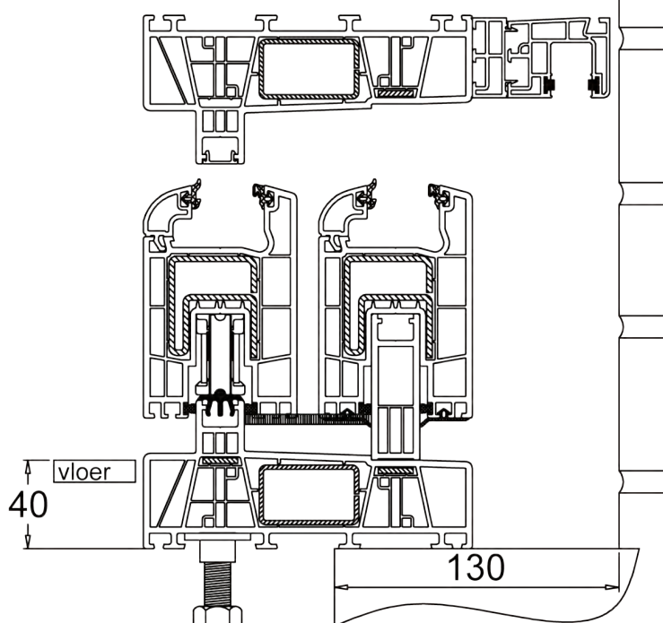
AD150 met rolluik en dunne schuifhor
