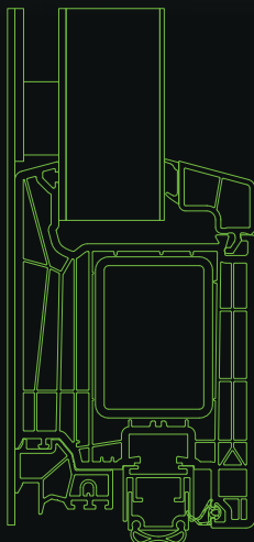
Vleugeloverdekkend paneel Panneau de porte cache-ouvrant
