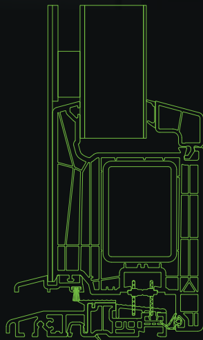
Vleugeloverdekkend paneel Panneau de porte cache-ouvrant
