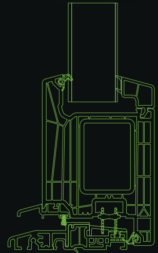
Standaard paneel Panneau de porte standard
